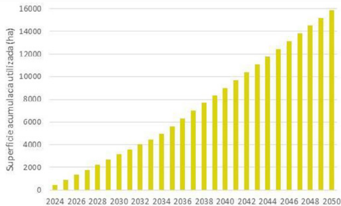
Figura 7-14. Superficie de suelo acumulada en hectáreas requerida para la explotación de uranio necesaria para el funcionamiento de las cuatro centrales nucleares incluidas en los escenarios
